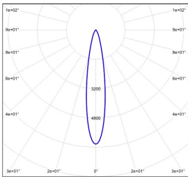
配光曲线@3000K数据
