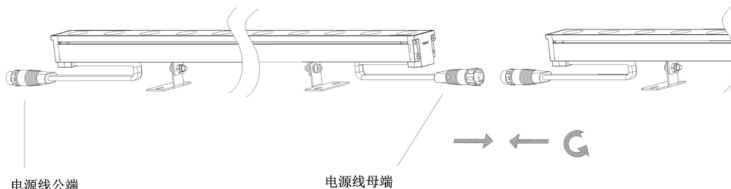
MT系列（DMX512调光）接线示意图
