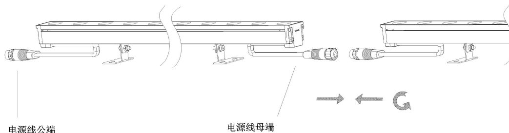
ET系列（ON/OFF）接线示意图
