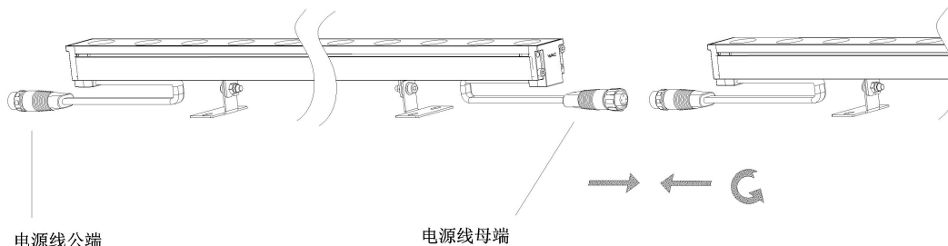
DT系列（0-10V调光）接线示意图
