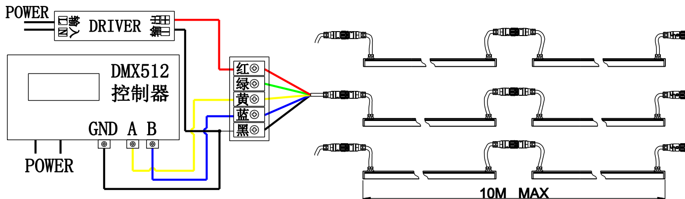
灯带接线示意图
