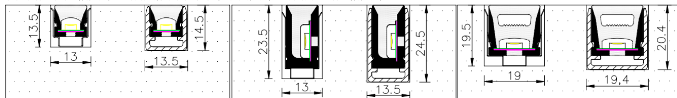
① 1010 灯带卡扣安装
